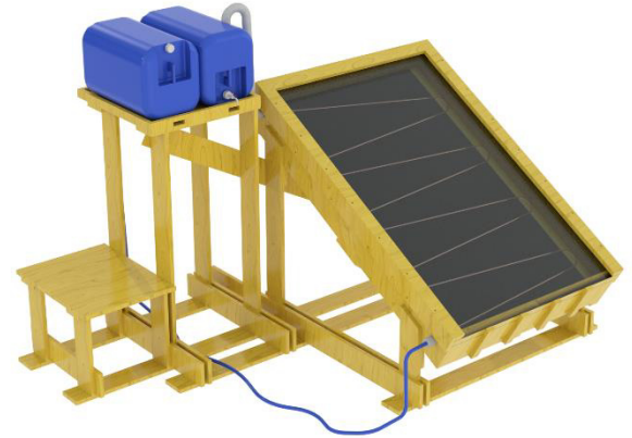
Computermodell der entwickelten SoWaDi-Anlage
